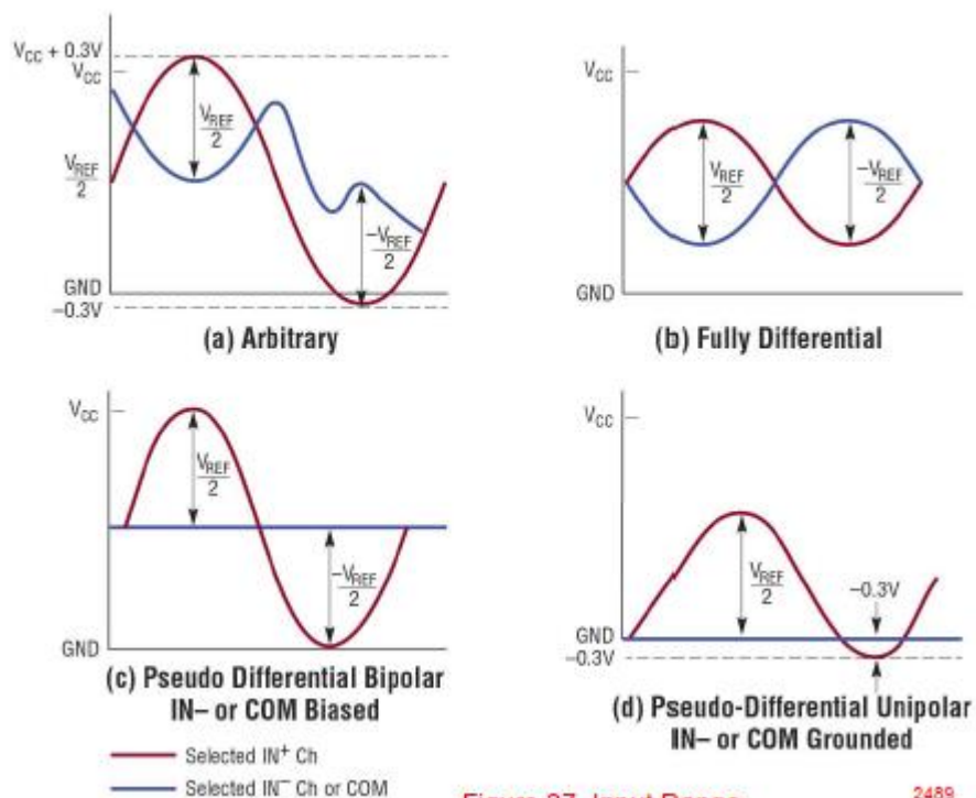
Figure 27. Input Range
