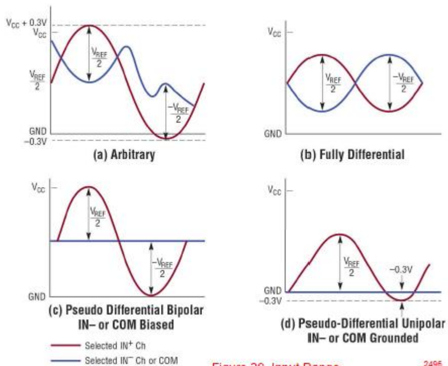
Figure 29. Input Range
