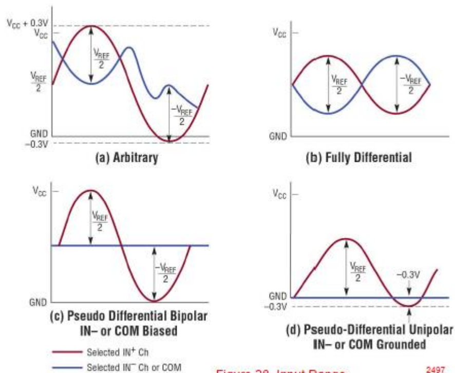
Figure 28. Input Range
