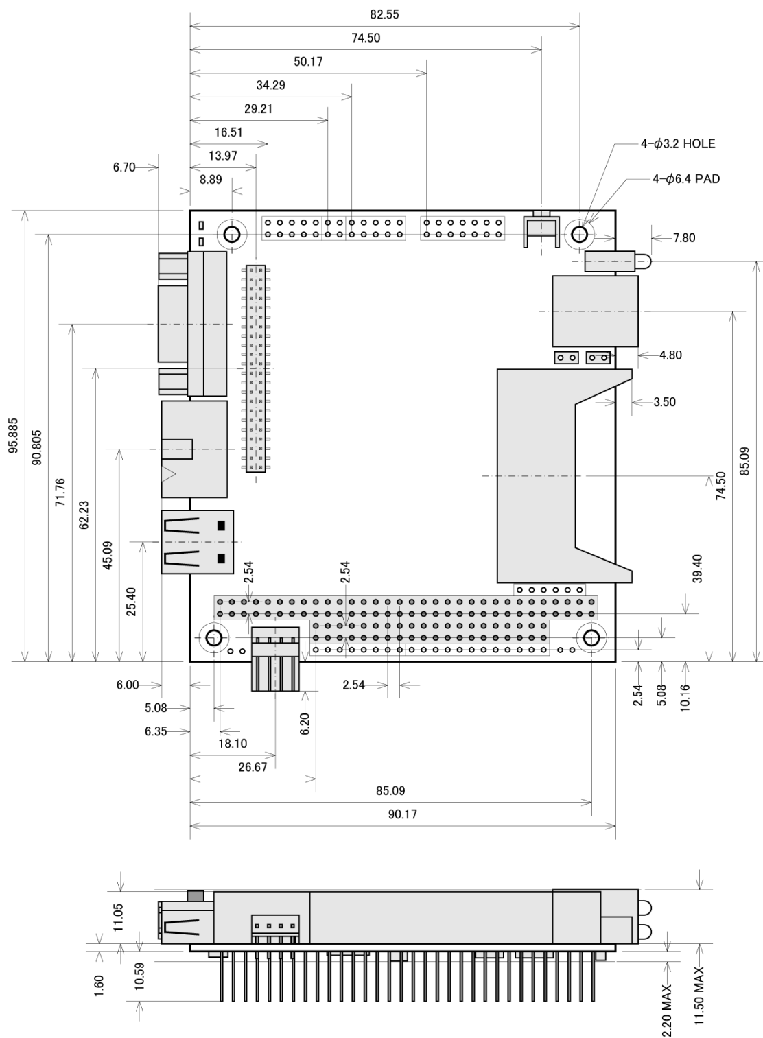
図1. 変更前の Armadillo-9 寸法図
