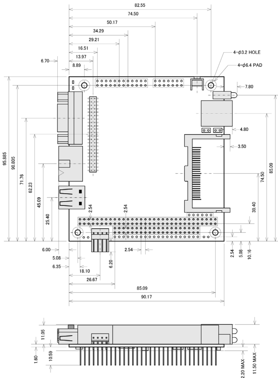
図2. 変更後の Armadillo-9 寸法図
