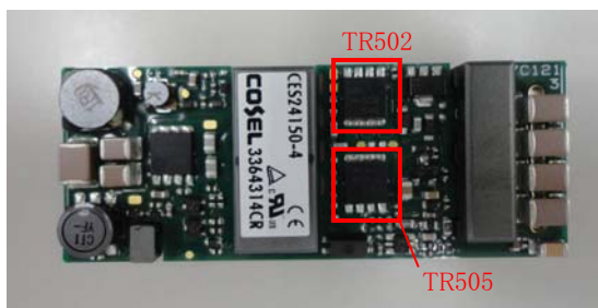
図1 表面、部品実装位置
