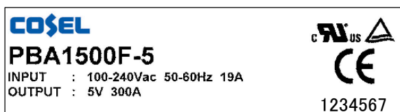
図1.1 現行品(出力電力300W以上)
