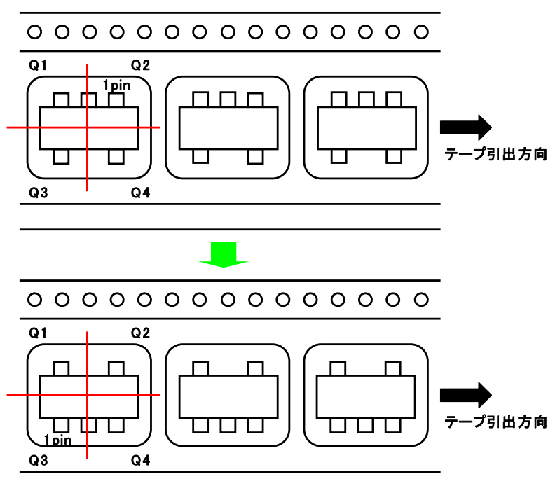
図 1. テープポケット内製品配置について
