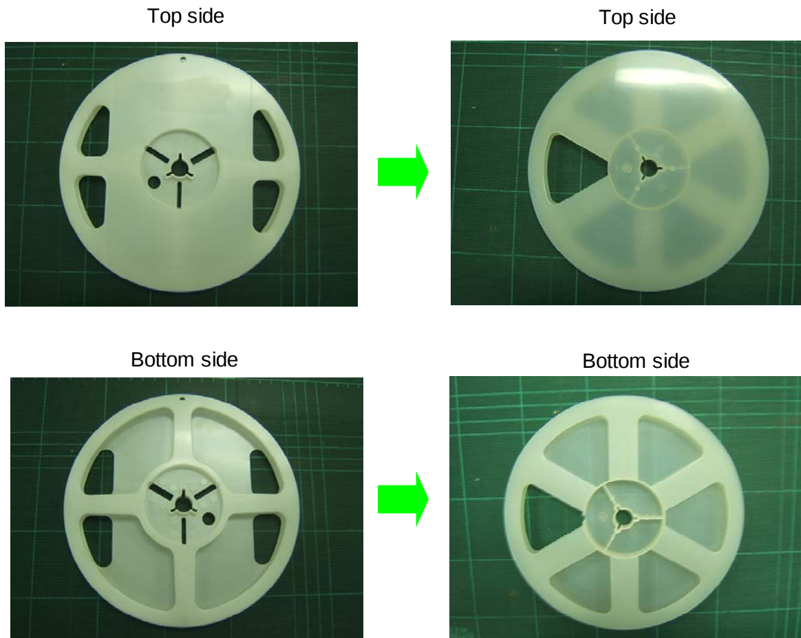
図 1、リール外観
