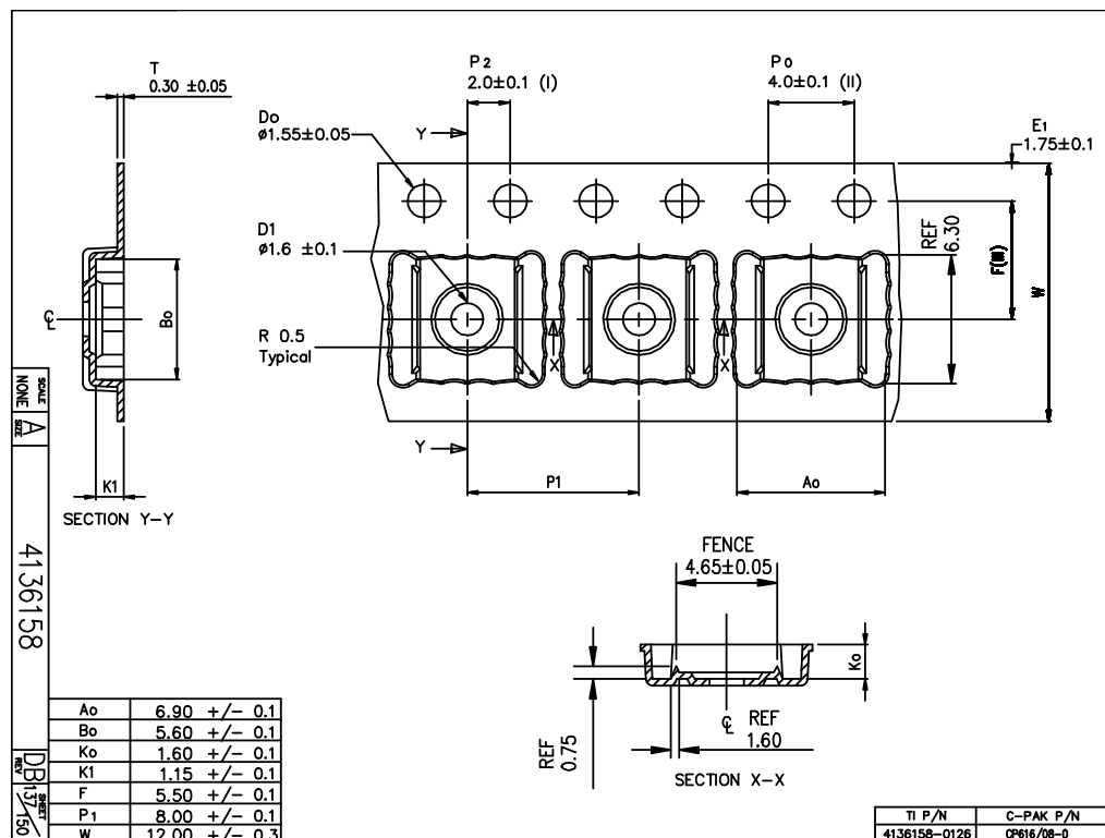
図2 変更後キャリアテープ外形寸法図(部材型番：4136158-0126)
