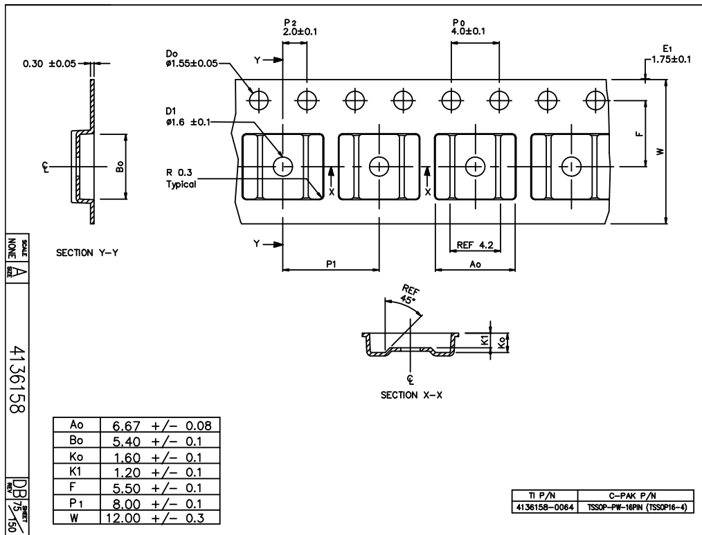
図1 現行キャリアテープ外形寸法図(部材型番：4136158-0064)
