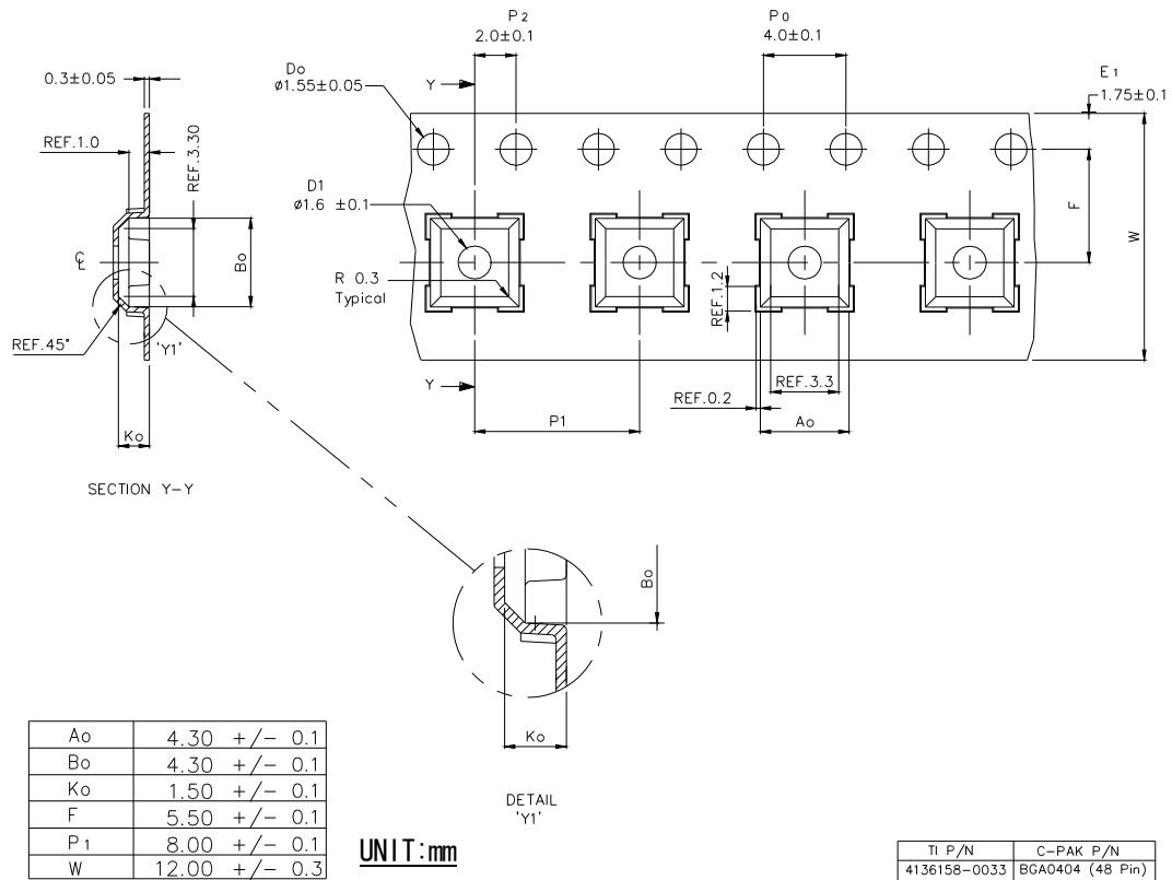
図1 現行キャリアテープ外形寸法図(部材型番：4136158-0033)
