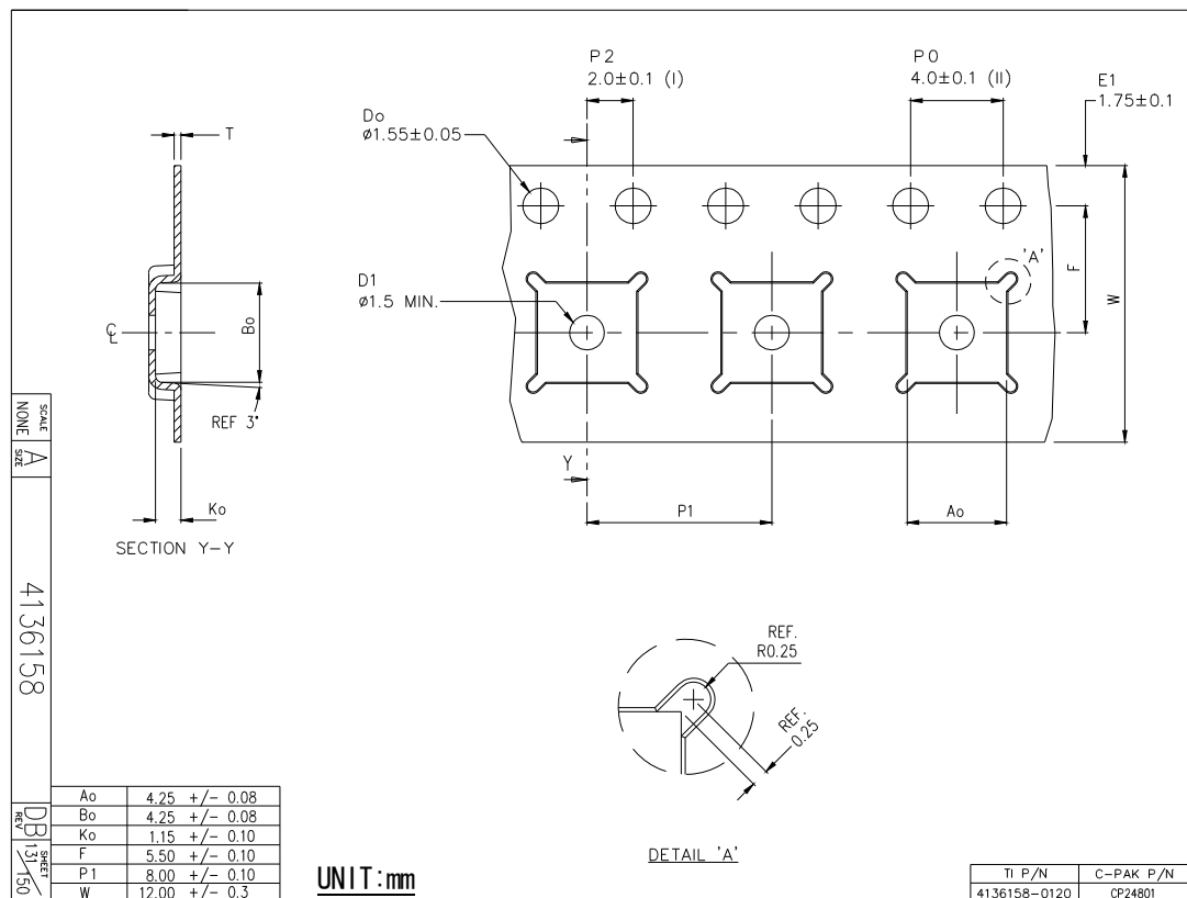
図2 変更後キャリアテープ外形寸法図(部材型番：4136158-0120)
