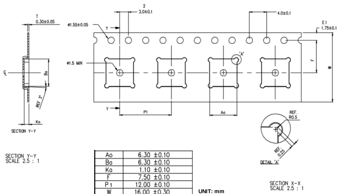
図2 変更後キャリアテープ寸法図
