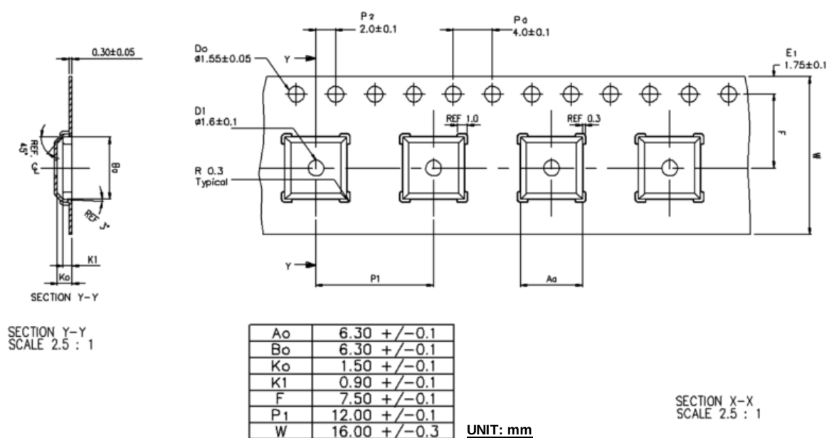
図1 現行キャリアテープ寸法図
