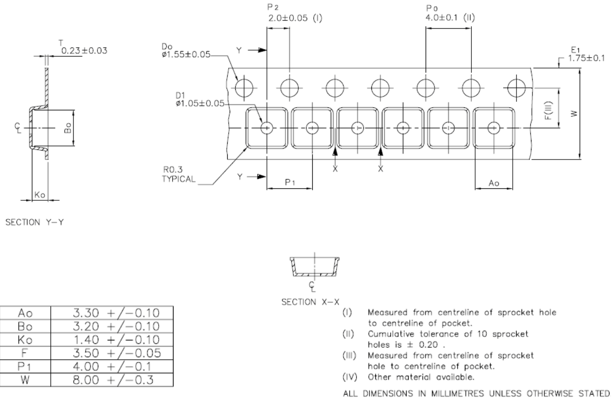
図1 変更後キャリアテープ寸法図 (C-PAK OT566)
