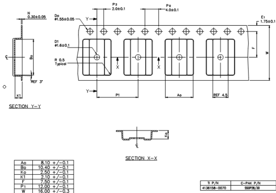
図1 変更後キャリアテープ寸法(部材番号: 4136158-0070)
